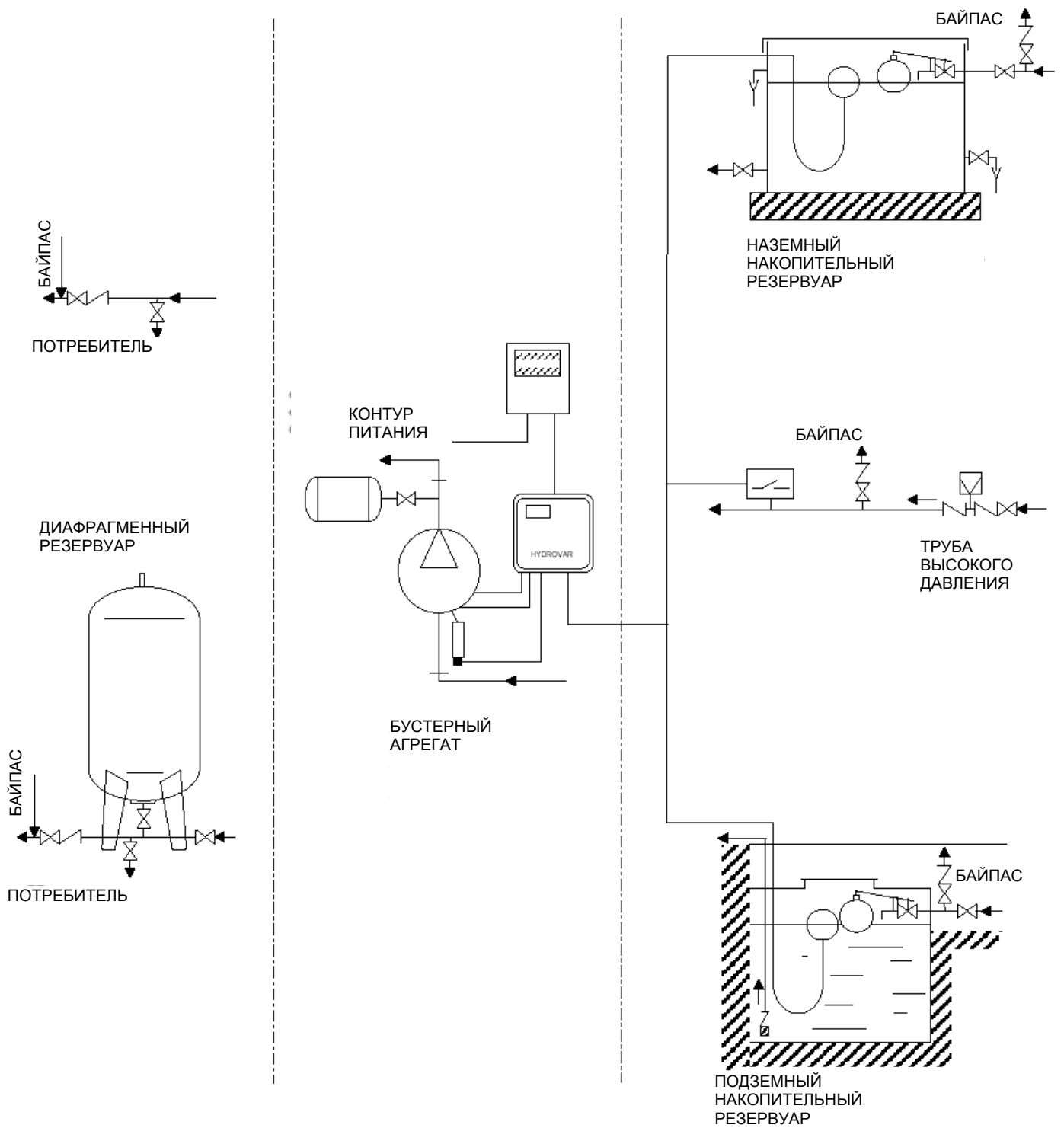
РИС. 3: ТИПИЧНАЯ СХЕМА УСТАНОВКИ (GHV10/...)
